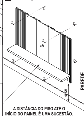
04 FIXAÇÃO DO PAINEL NA PAREDE
