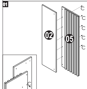
02 AO PARAFUSAR ESCOLHA A LARGURA DO SEU PAINEL
