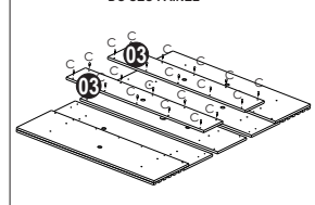
03 FIXAÇÃO DO PAINEL NA PAREDE
